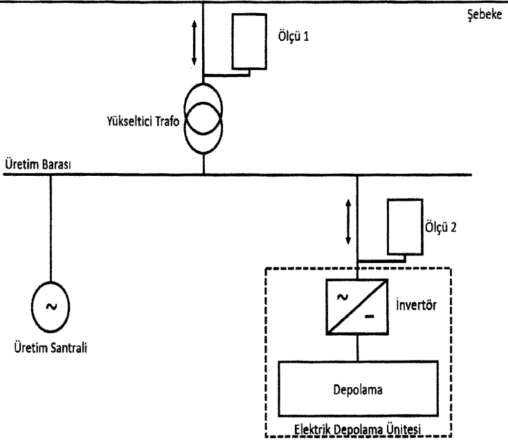
EK-1: Depolamalı Elektrik Üretim Tesisi ile Üretim Tesisine Bütünleşik Elektrik Depolama Ünitesine Ait Bağlantı Konfigürasyonu
